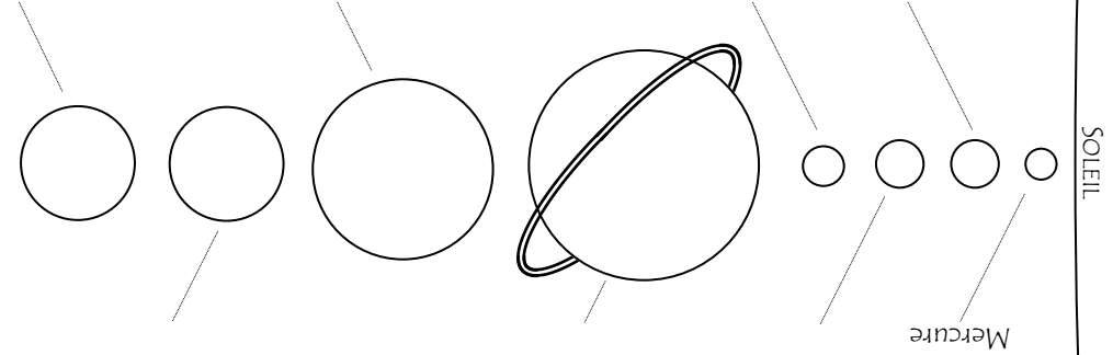
SCHEMA REPRESENTANT LES PLANETES DU SYSTEME SOLAIRE (SANS ECHELLE)
